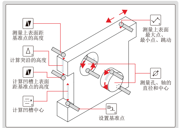
一维测量
